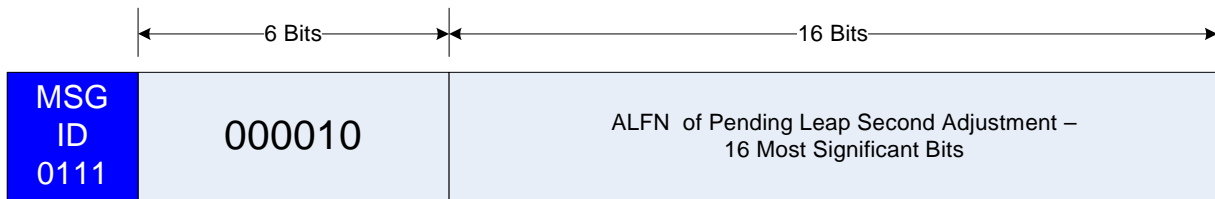
Figure 4-14: Format of SIS Parameter Message Index 2
