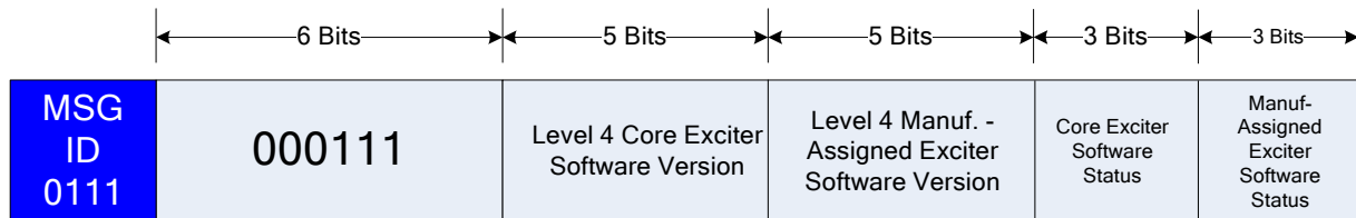
Figure 4-19: Format of SIS Parameter Message Index 7
