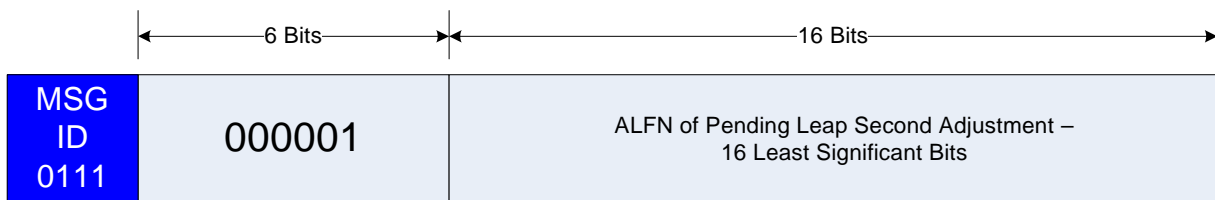
Figure 4-13: Format of SIS Parameter Message Index 1
